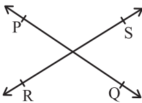
(i) ಭೇದಿಸುವ ರೇಖೆಗಳು
