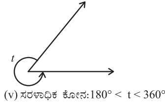
ಚಿತ್ರ : 6.1 ಕೋನದ ವಿಧಗಳು
