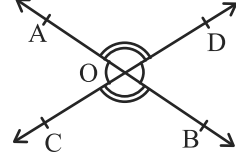
ಚಿತ್ರ 6.8 ಶೃಂಗಾಭಿಮುಖ ಕೋನಗಳು
