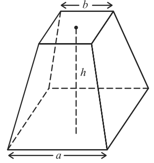
ಚಿತ್ರ 5.1 : ಭಿನ್ನಗ್ರ ಪಿರಮಿಡ್
