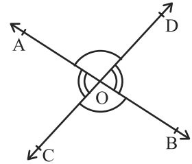
ಚಿತ್ರ 6.4 ಶೃಂಗಾಭಿಮುಖ ಕೋನಗಳು
