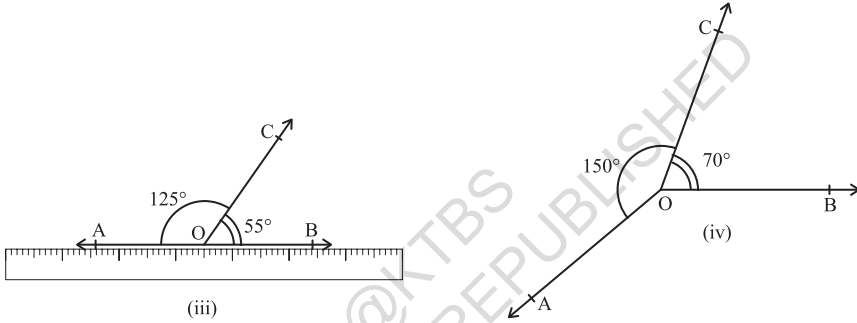
ಚಿತ್ರ : 6.7 ವಿವಿಧ ಅಳತೆಗಳುಳ್ಳ ಪಾರ್ಶ್ವಕೋನಗಳು
